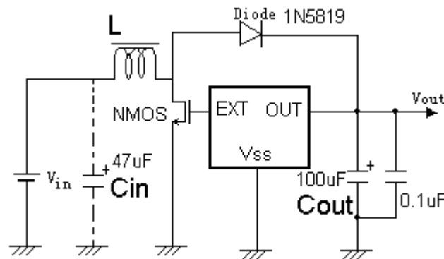
图二: TP8356X 典型应用电路
